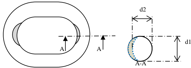
Rysunek nr 5. Wewnętrzne zużycie ogniwa
