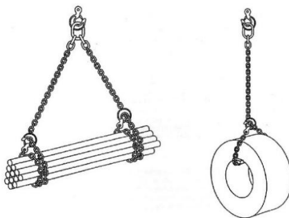
Rysunek nr 1. Zawieszanie z obwiązywaniem pętli przesuwną
